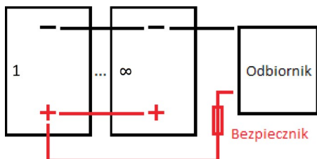
Rys.3. Schemat szeregowego połączenia akumulatorów
