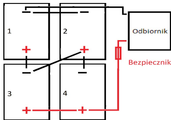
Rys.4. Schemat szeregowo-równoległego połączenia akumulatorów
